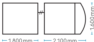
Geteiltes Gehäuse
